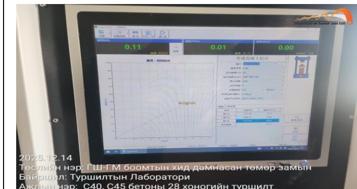
C40, C45 ангилалын бетоны 28 хоногийн туршилт
