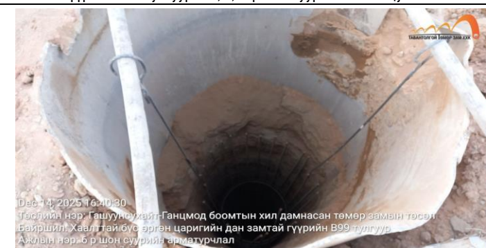
Гүүрийн B99 тулгуурын 6-р шон суурийн арматурчлал байрлуулах
